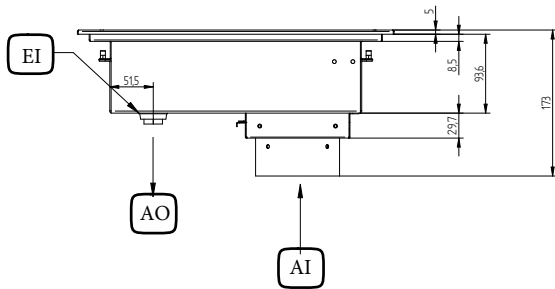
Boční
